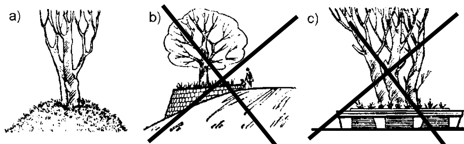
a) pozostawiony ścięty stożek z gruntu, ochraniający korzenie drzewa b) ścianka podporowa z kamienia wokół drzewa pozostawionego na skarpie c) ścianka oporowa dostosowana do odpoczynku podróżnych przez wykonanie ławki na jej górnej powierzchni
