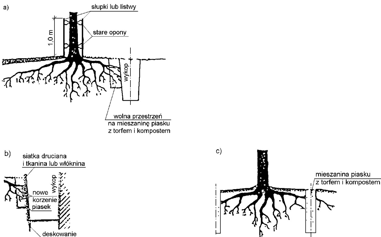
a) przekrój ogólny, b) szczegół wykopu, c) wstępna faza zabezpieczenia, wykonywana najlepiej rok przed właściwym wykopem
