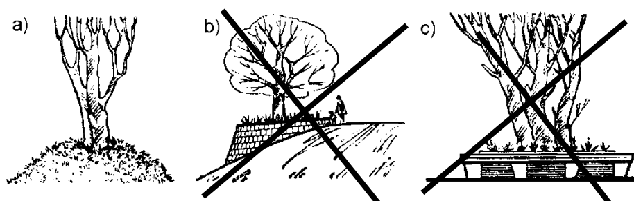
a) pozostawiony ścięty stożek z gruntu, ochraniający korzenie drzewa b) ścianka podporowa z kamienia wokół drzewa pozostawionego na skarpie c) ścianka podporowa dostosowana do odpoczynku podróżnych przez wykonanie ławki na jej górnej powierzchni
