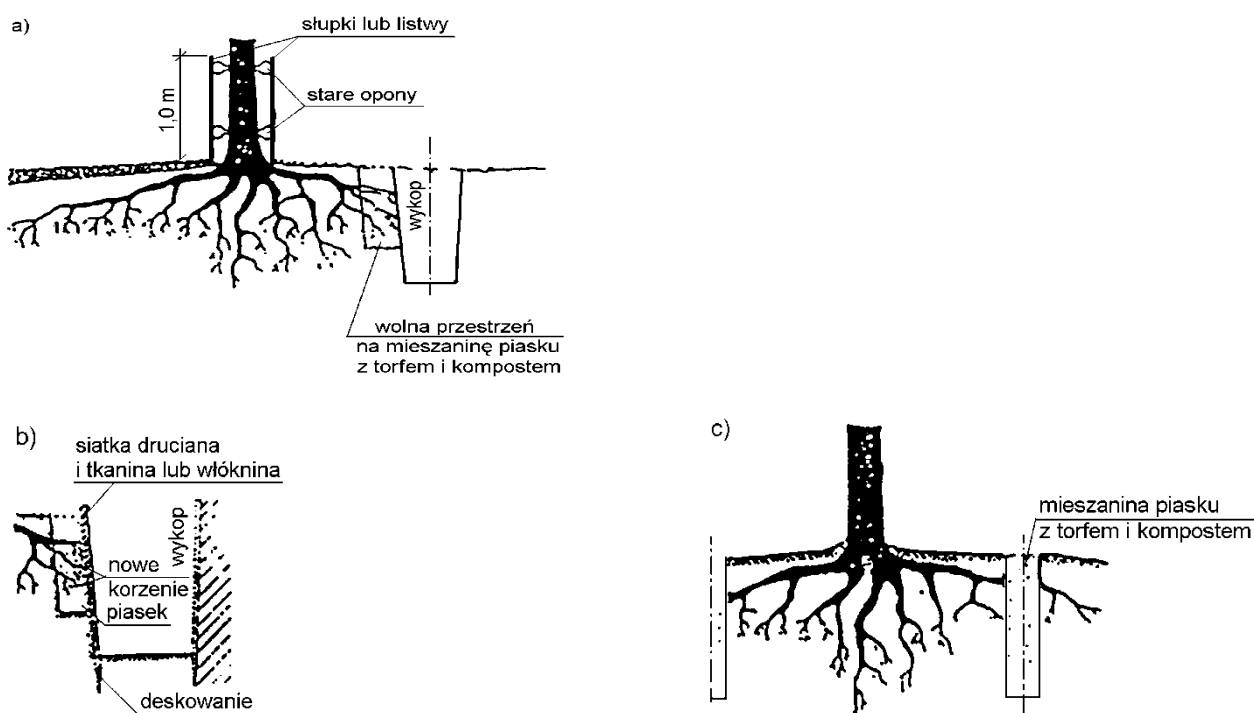
a) przekrój ogólny, b) szczegół wykopu, c) wstępna faza zabezpieczenia, wykonywana najlepiej rok przed właściwym wykopem
