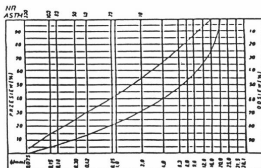
Rys.8. Krzywe graniczne uziarnienia mieszanki mineralnej 0/20mm do mieszanki z betonu asfaltowego półściśłego.
