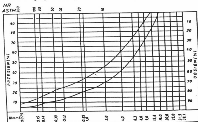
Tablica Nr 13 Wymagania dla mieszanki betonu asfaltowego 0/20 mm półcisłego
