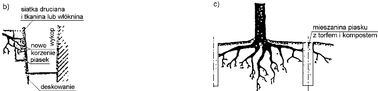
a) przekrój ogólny, b) szczegół wykopu, c) wstępna faza zabezpieczenia, wykonywana najlepiej rok przed właściwym wykopem
