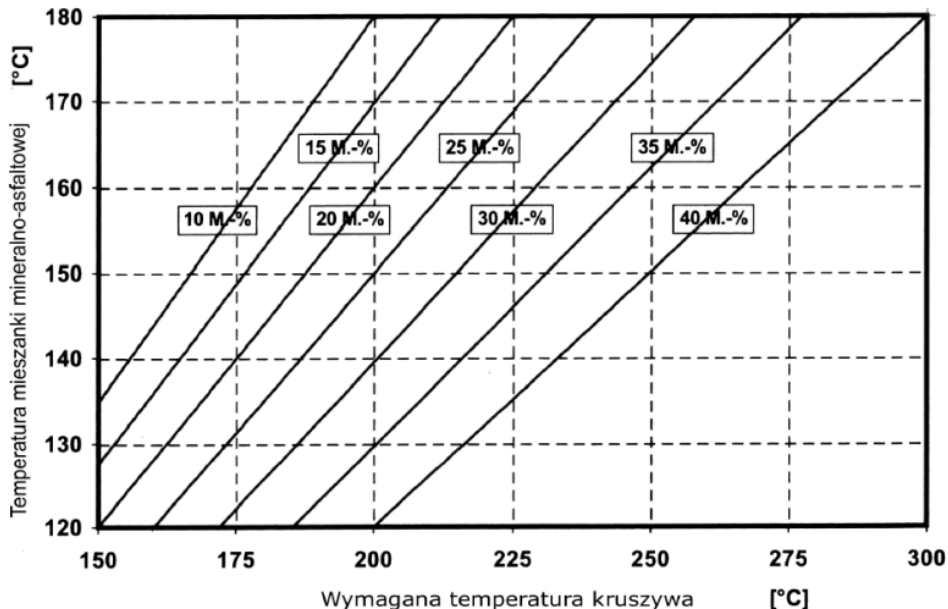
Tablica - Korekta temperatury produkcji w zależności od wilgotności granulatu asfaltowego.
