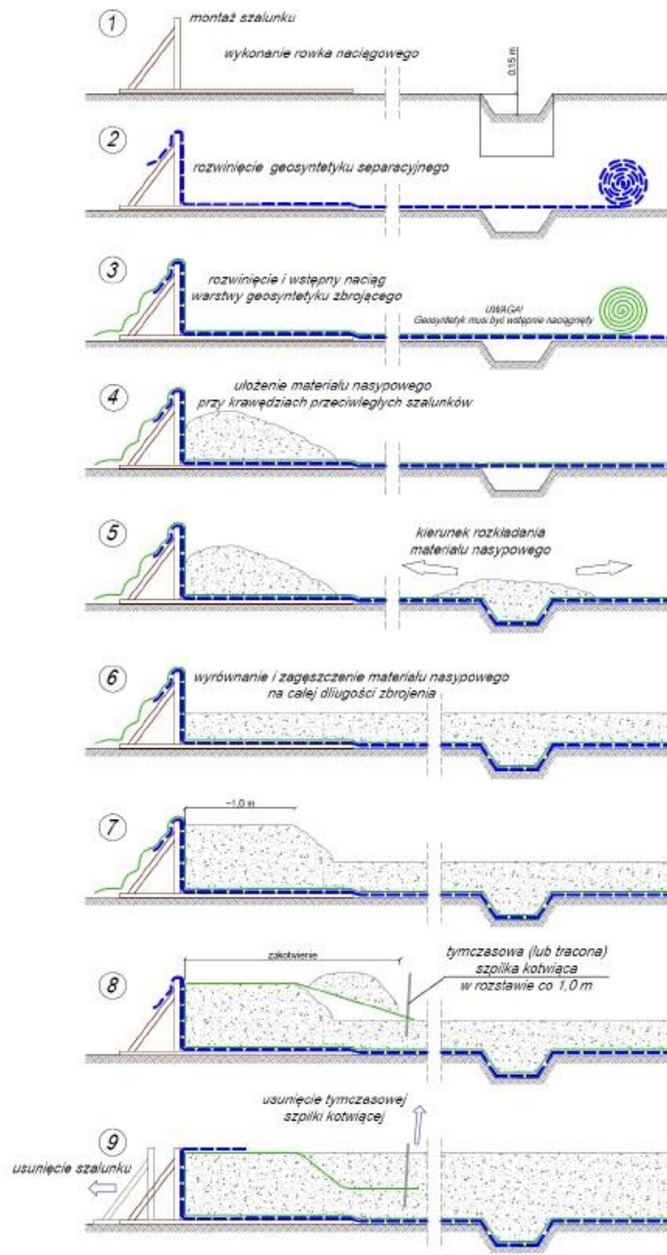
Rys. Przykładowy schemat ułożenia warstw geosyntetycznych
