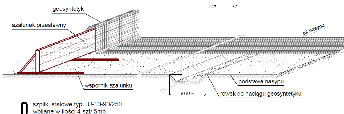
Rys. Przykładowy schemat wykonania szalunków oraz rowu naciągowego
