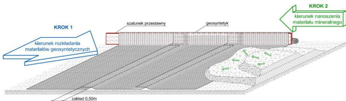
Rys. Przykładowy schemat układania materiałów geosyntetycznych oraz układania warstw materiału mineralnego
